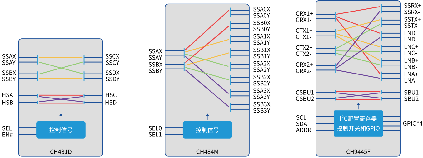
应用框图 \ Block Diagram
